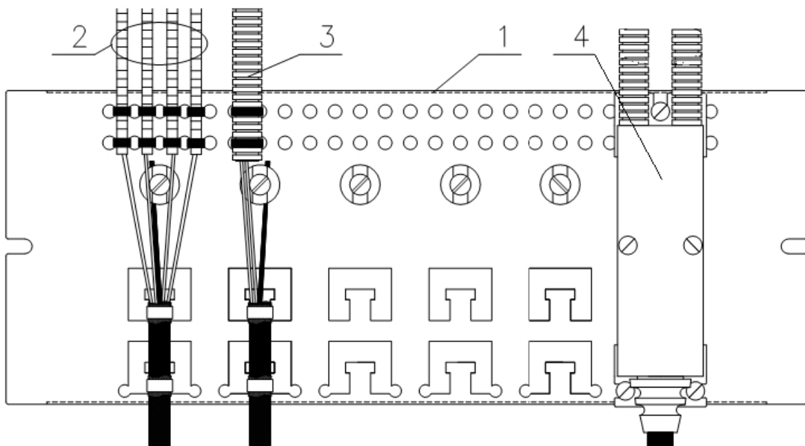
Rys.1: Mocowanie kabli na listwie rozszycia. Elementy: [1]-listwa rozszycia; [2]-tuba ochronna; [3]-peszel; [4]- rozdzielacz
